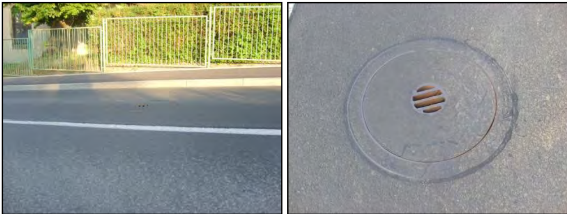
Abb. 29 Lärmarme Schachteindeckung (Beispiel Dresden)
